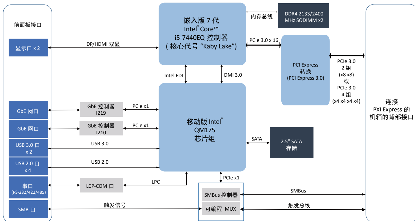
PXIe-63977架构图
