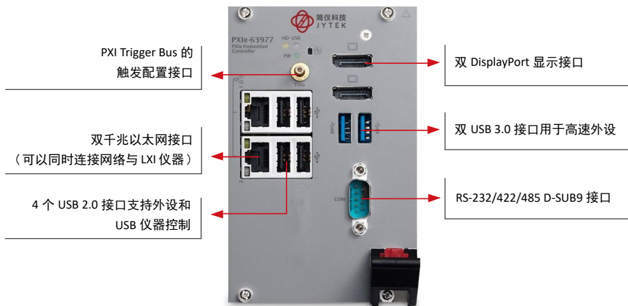
PXle-63977 前面板
