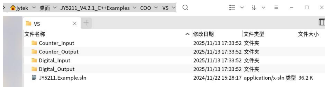
图 5-16 C00 范例
