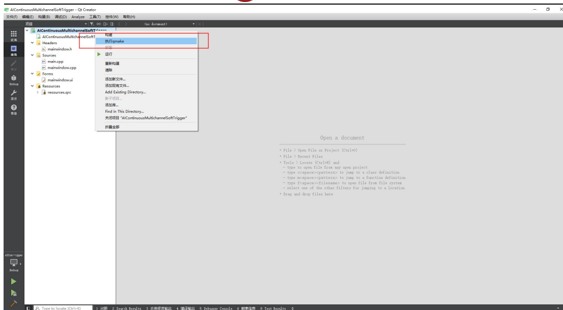
图 8-36 qmake
