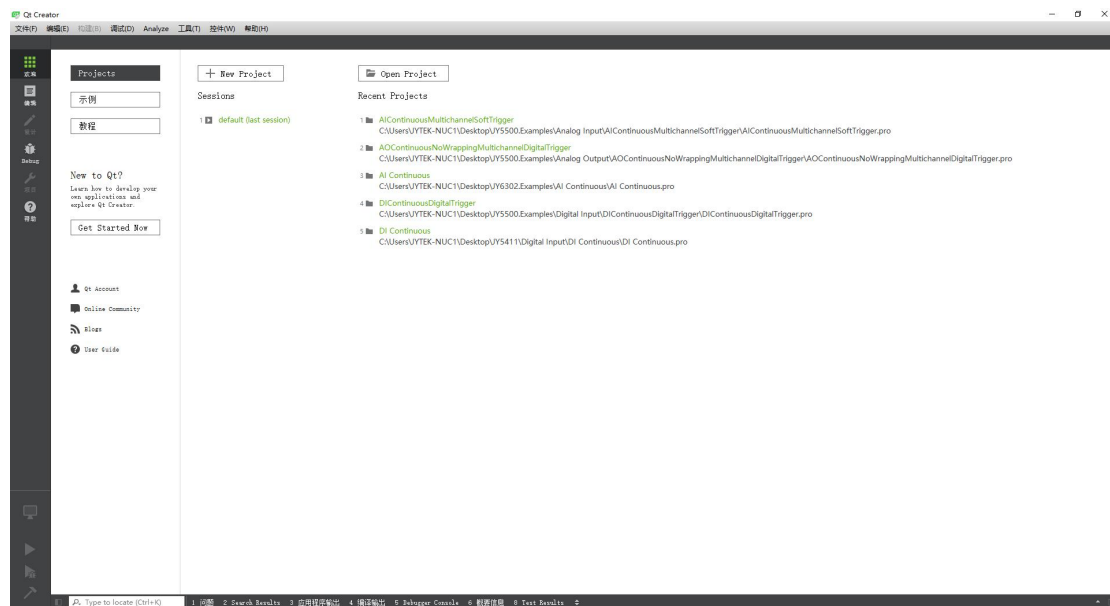
图 8-14 Qt 界面
